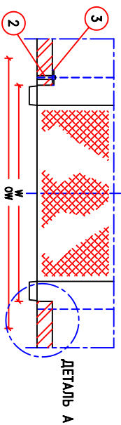
РАЗРЕЗ А-А
